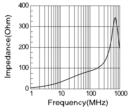
RH-3.5x6.0x0.8
