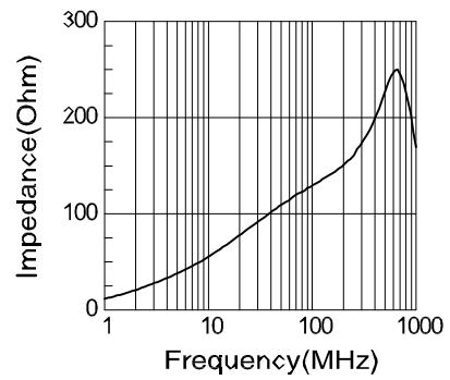
RH-3.5x8.0x0.8
